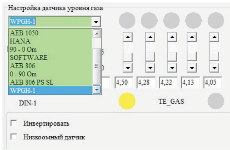
WPGH-1 level sensor setting in Tegas software Установка датчика WPGH-1 в программе Tegas
