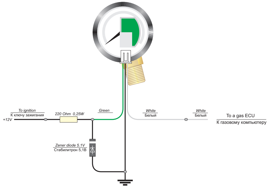
Sensor connection scheme Схема подключения датчика
